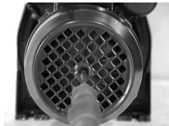
Para evitar bloqueo del sello mecánico, hacer girar el eje a través del ventilador antes de la puesta en marcha o después de una inutilización prolongada!
